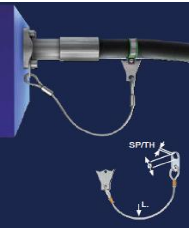
Kiinnitys SAE-laippaan
