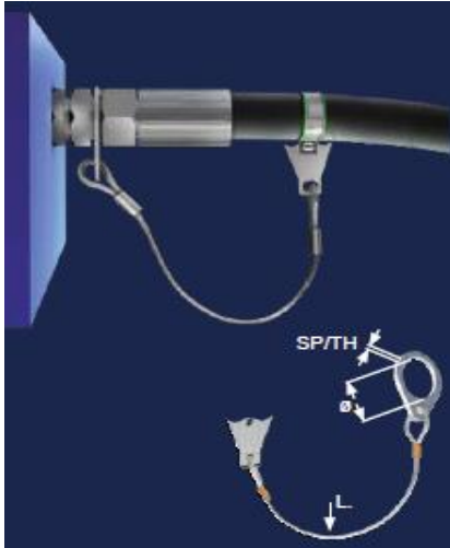
Kiinnitys nippaan
